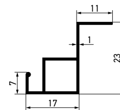
Profil 23 mm za fiksni komarnik Bela 9016 - 6 m
