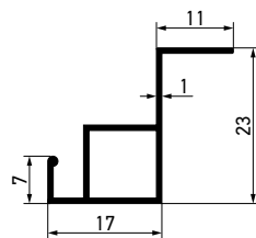
Profil 23 mm za fiksni komarnik Braon 8017 - 6 m
