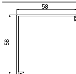
F60 pokrivni profil za stub skretnicu 90° - 6 m Antracit RAL 7016
