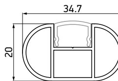
F40 Classic vertikalni profil 20×34.7 mm - 6 m Antracit RAL 7016
