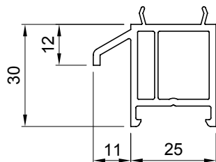
Podštok 30×25 mm
