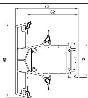
T prečka 76 mm MD
