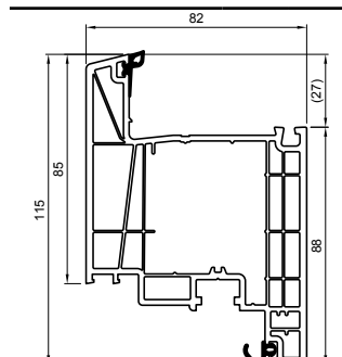
Krilo vrata 82 mm - unutrašnje
