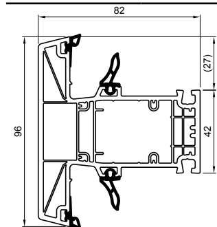
T prečka 82 mm MD Antracit
