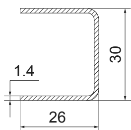
Ojačanje za štok MD, krilo i T prečku MD - 1.4 mm 6m 263026.14 8.65€
