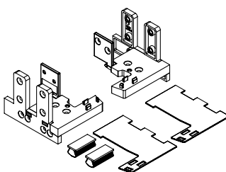
Čepovi za alu prag R+L
