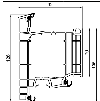
Krilo vrata - spoljašnje
