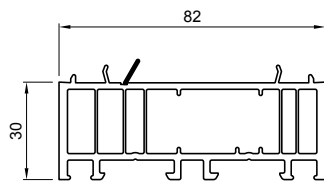
Proširenje 82×30 mm
