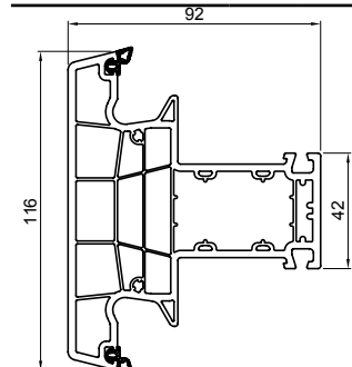
T prečka
