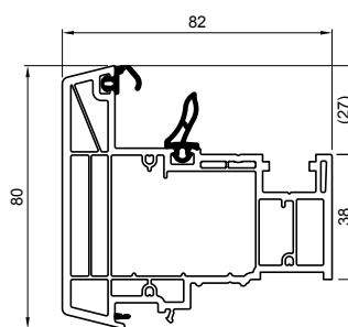
Lažna prečka 82 mm MD
