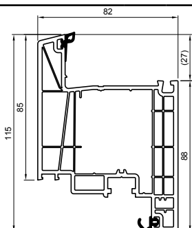
Krilo vrata 82 mm - unutrašnje
