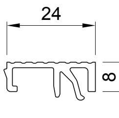
Pokrivni profil za prag 82 mm
