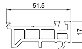
Adapter za fix
