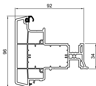
Lažna prečka
