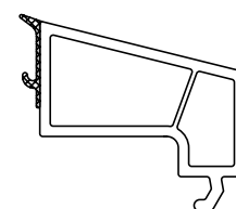
Lajsna za staklo 24 mm
