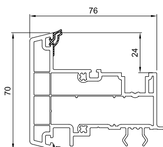
Lažna prečka 76 mm AD
