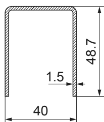
Ojačanje za krilo vrata 1.5 mm 6m 484048.15 24.00€
