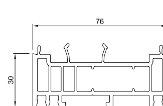
Proširenje 76x30 mm
