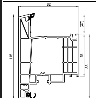
Krilo vrata 82 mm - spoljašnje Antracit
