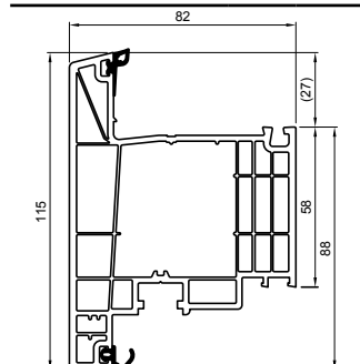
Krilo vrata 82 mm - spoljašnje
