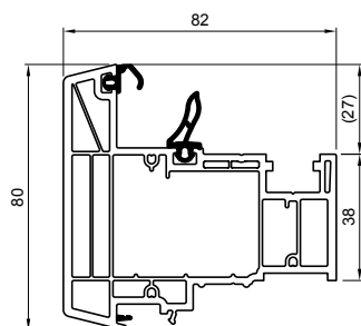
Lažna prečka 82 mm MD
