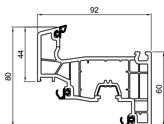
Krilo
