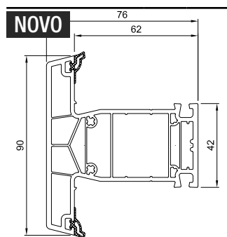
T prečka 76 mm AD
