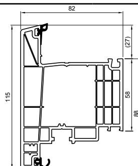
Krilo vrata 82 mm - spoljašnje
