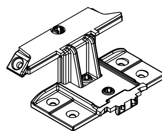
Spojnica za T prečku
