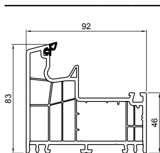
Štok
