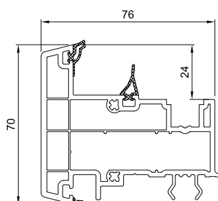
Lažna prečka 76 mm MD
