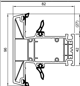
T prečka 82 mm MD
