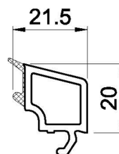
Lajsna za staklo 48 mm
