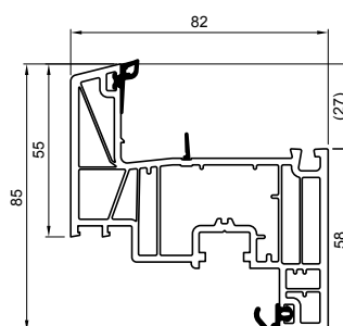
Krilo 82 mm - Antracit spolja
