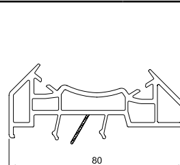
Adapter za varijabilnu skretnicu
