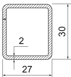
Ojačanje za štok MD i T prečku MD - 2 mm 6m 465002-074 31.15€
