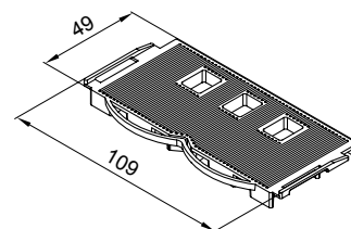
Osnovna kajla za štok
