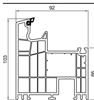
Štok veći
