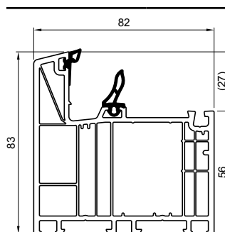
Štok veći 82 mm MD
