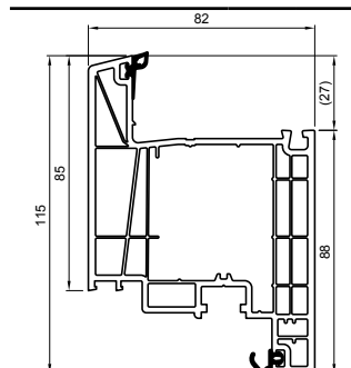
Krilo vrata 82 mm - unutrašnje Antracit
