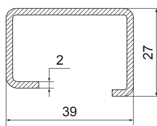
Ojačanje za krilo 2 mm 6m 465006-074 26.00€
