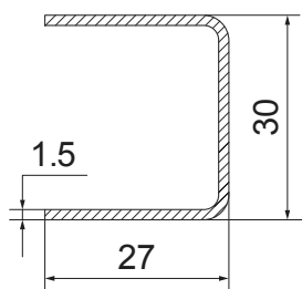
Ojačanje za štok MD, krilo i T prečku MD - 1.5 mm 6m 273027.15 9.70€
