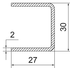
Ojačanje za štok MD, krilo i T prečku MD - 2 mm 6m 273027.20 13.50€
