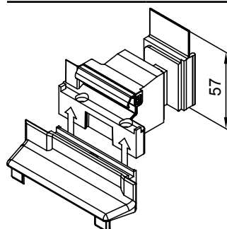
Čep za lažnu prečku
