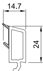
Lajsna za staklo 44 mm
