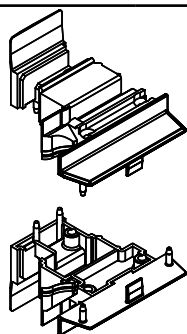
Čep lažne prečke
