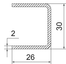
Ojačanje za štok MD, krilo i T prečku MD - 2 mm 6m 263026.20 USKORO
