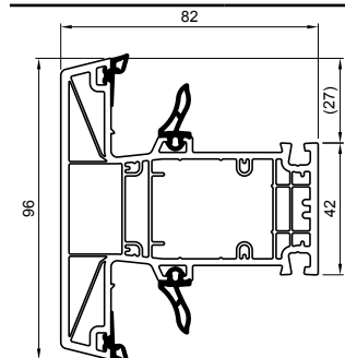
T prečka 82 mm MD
