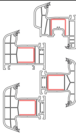
Ojačanje za laminirane profile
