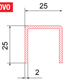
Ojačanje za laminirane profile
