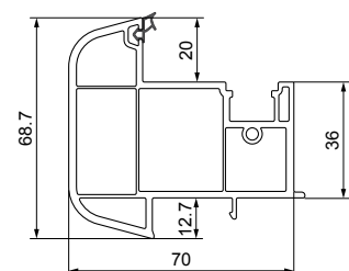
Lažna prečka 70 mm
