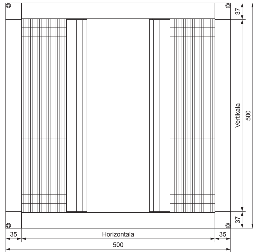
Dva zatvarajuća krila
