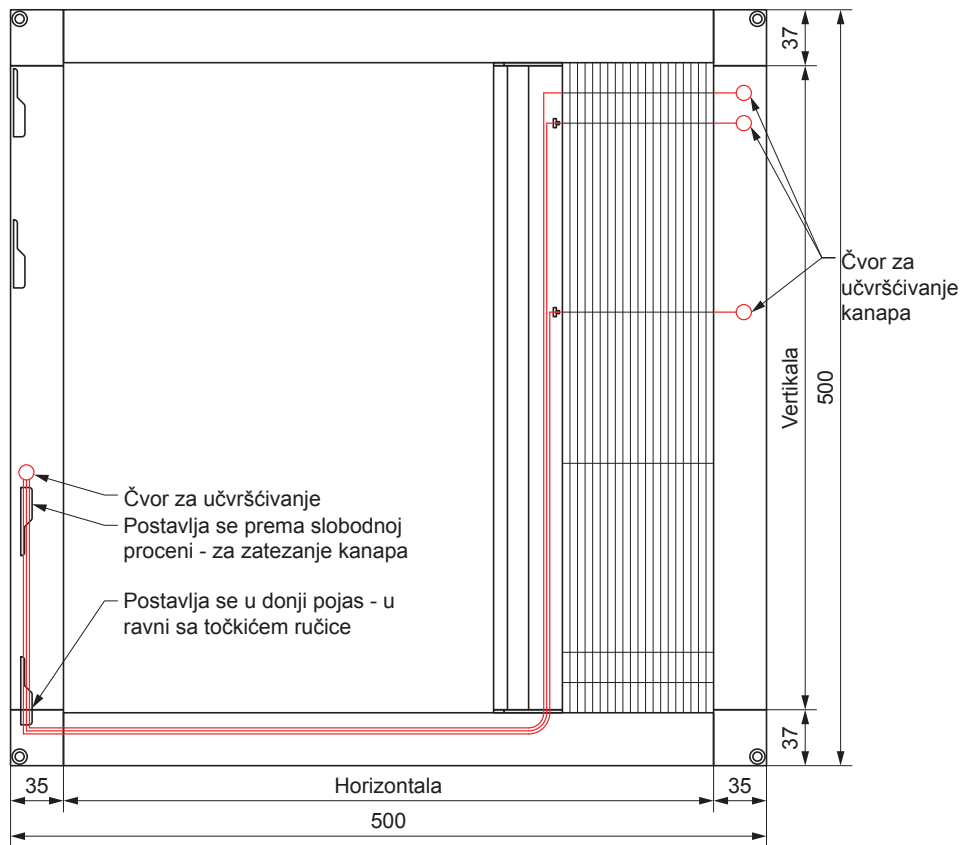
Šema postavljanja kanapa
